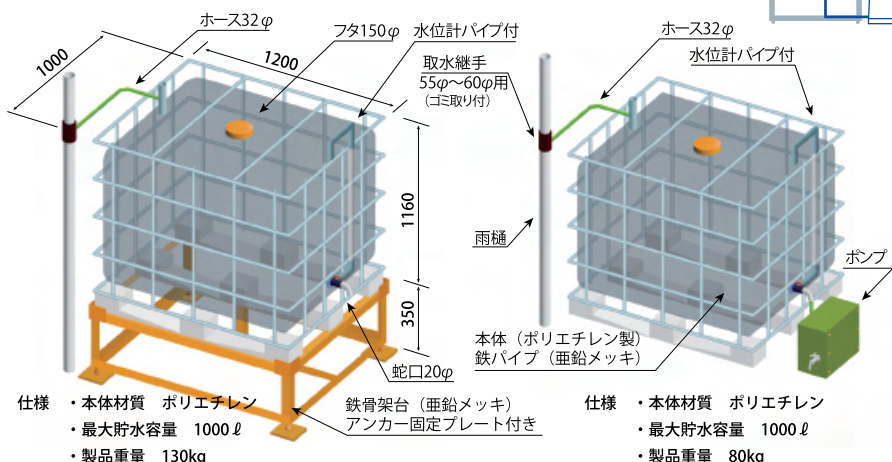
圧送手押しポンプと 浄水器の取付け例 →
